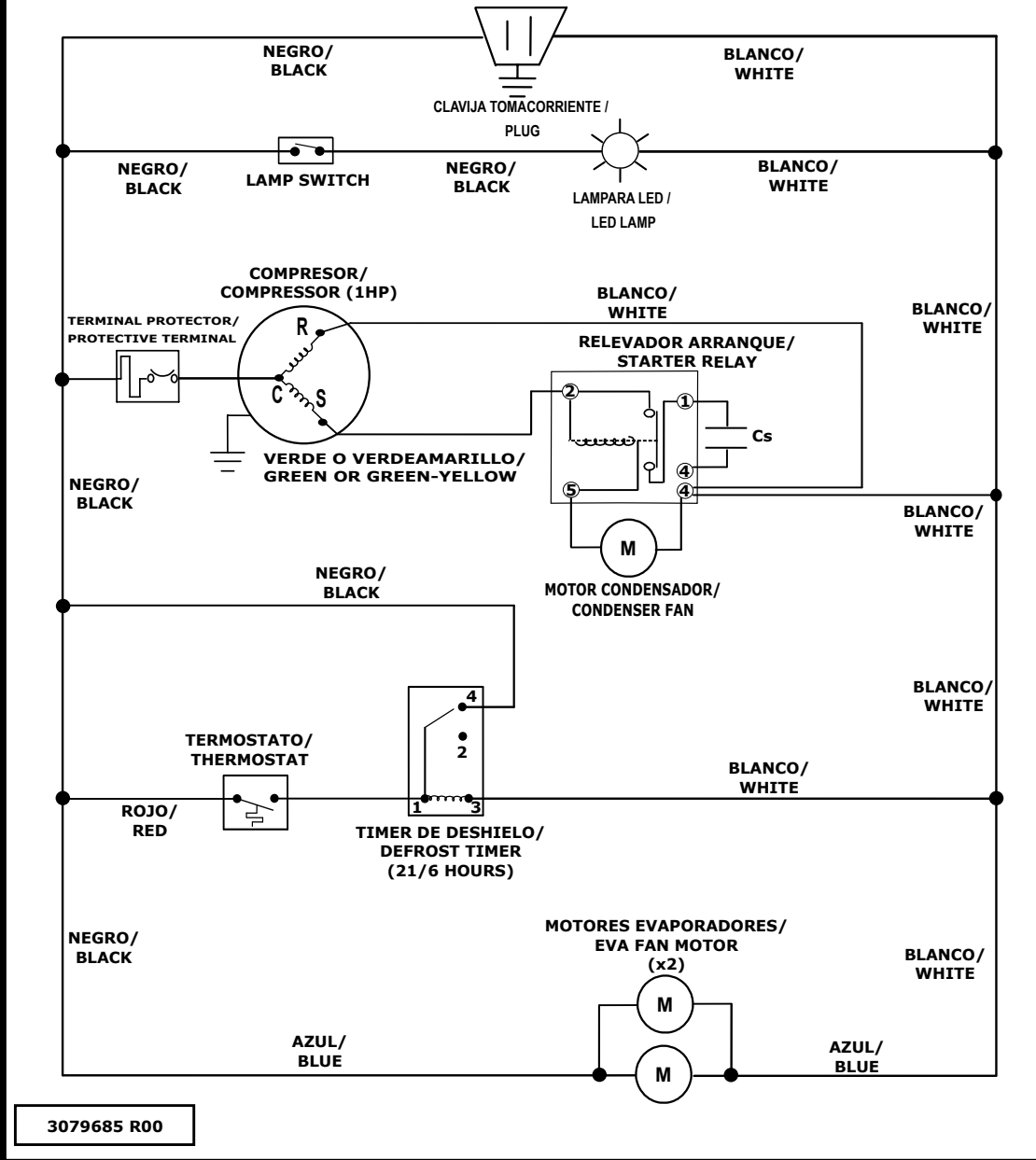
DIAGRAMA ELECTRICO UNIDAD INTEGRAL REFRIGERACION 127V 60Hz / ELECTRICAL DIAGRAM INTEGRAL UNIT REFRIGERATOR 127V 60Hz
