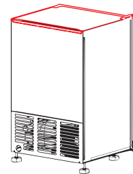
ENSAMBLE EVAPORADOR
